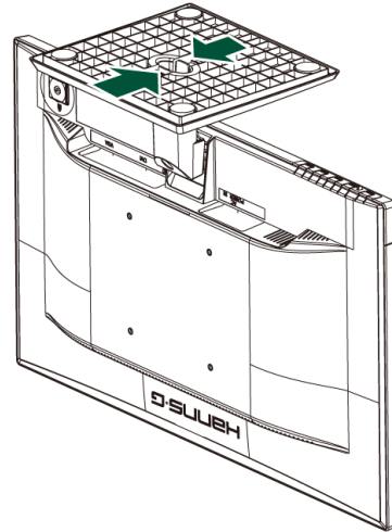
Фигура 1 Монтаж и демонтаж на основата
