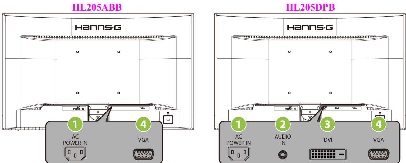
Figur 2. Tilslutning af kabler
