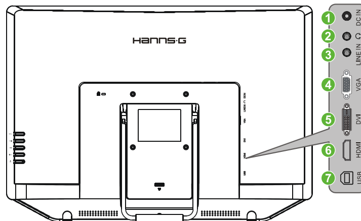
Figur 2. Tilslutning af kabler
