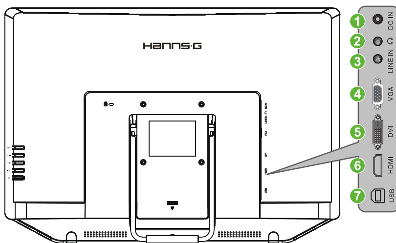
图二. 连接到 PC
