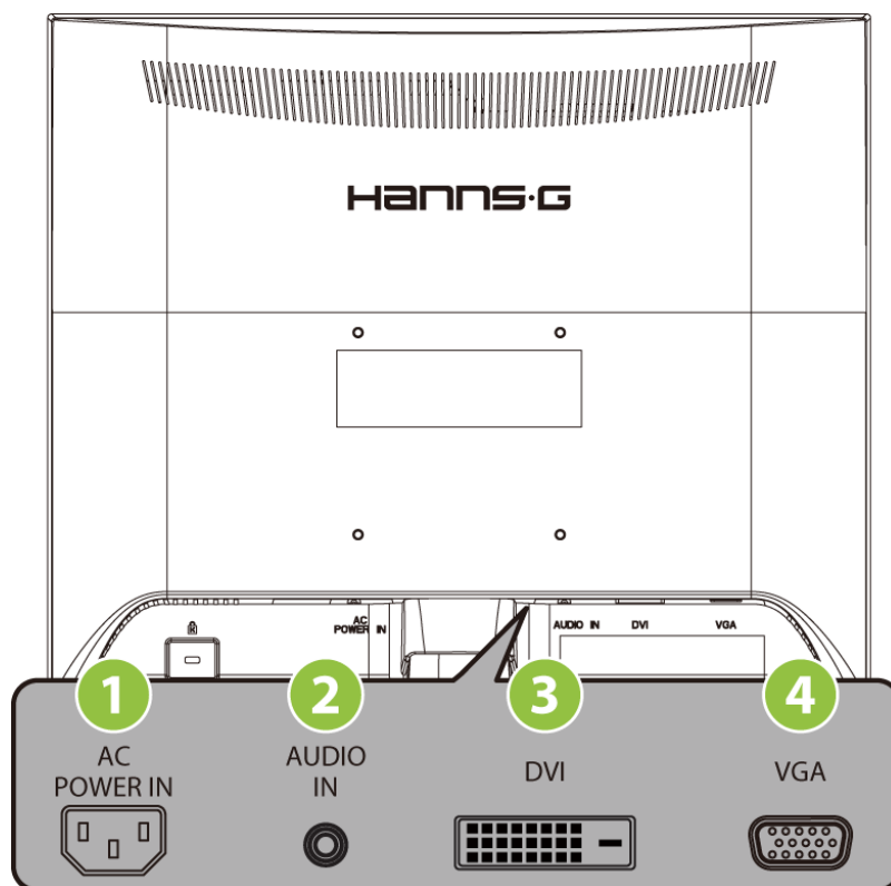
Рисунок 2: Подключение к ПК
