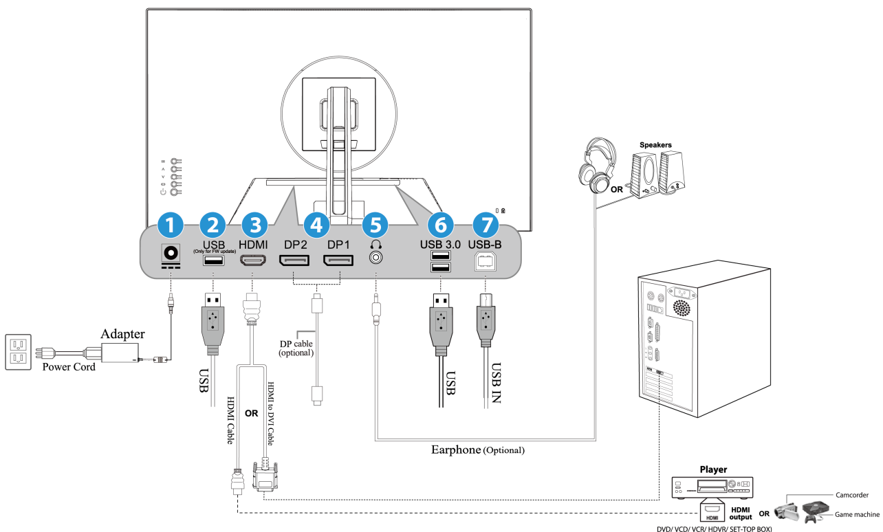
ABBILDUNG 2. ANSCHLISSEN AN EINEN PC
