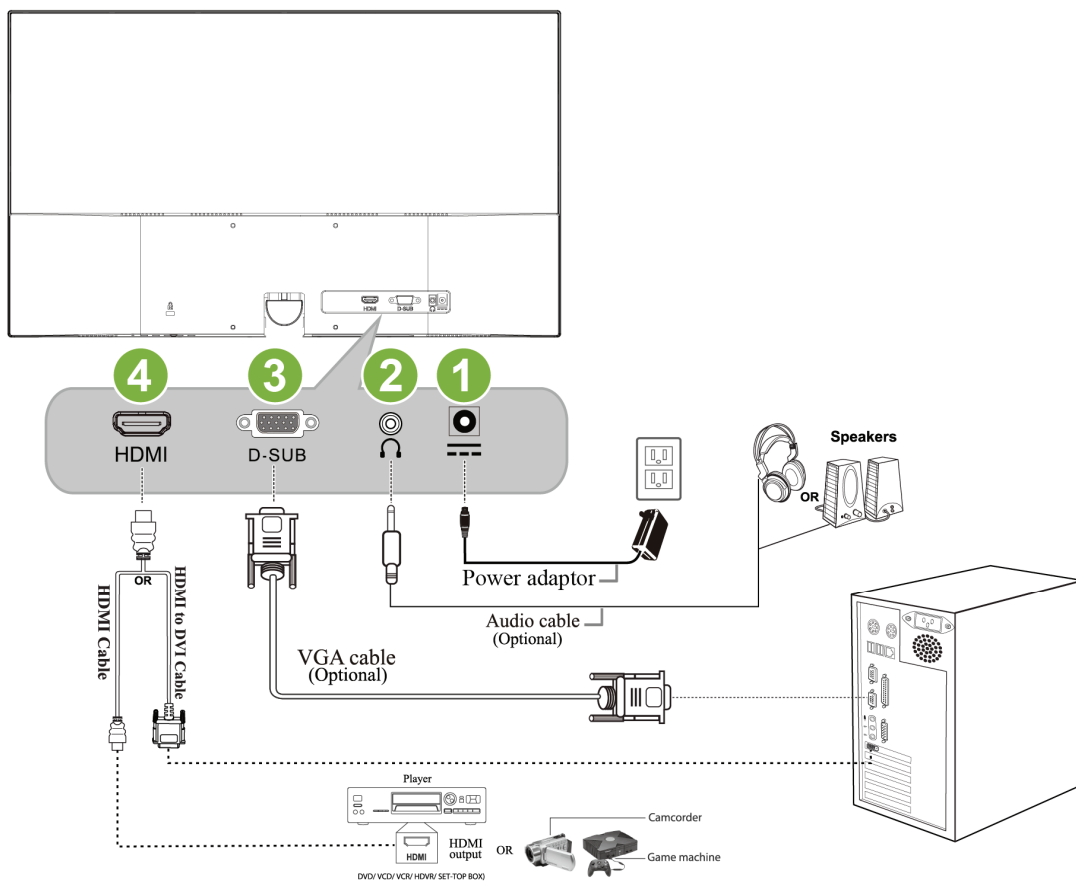
Figura 2. Conexión a un PC
