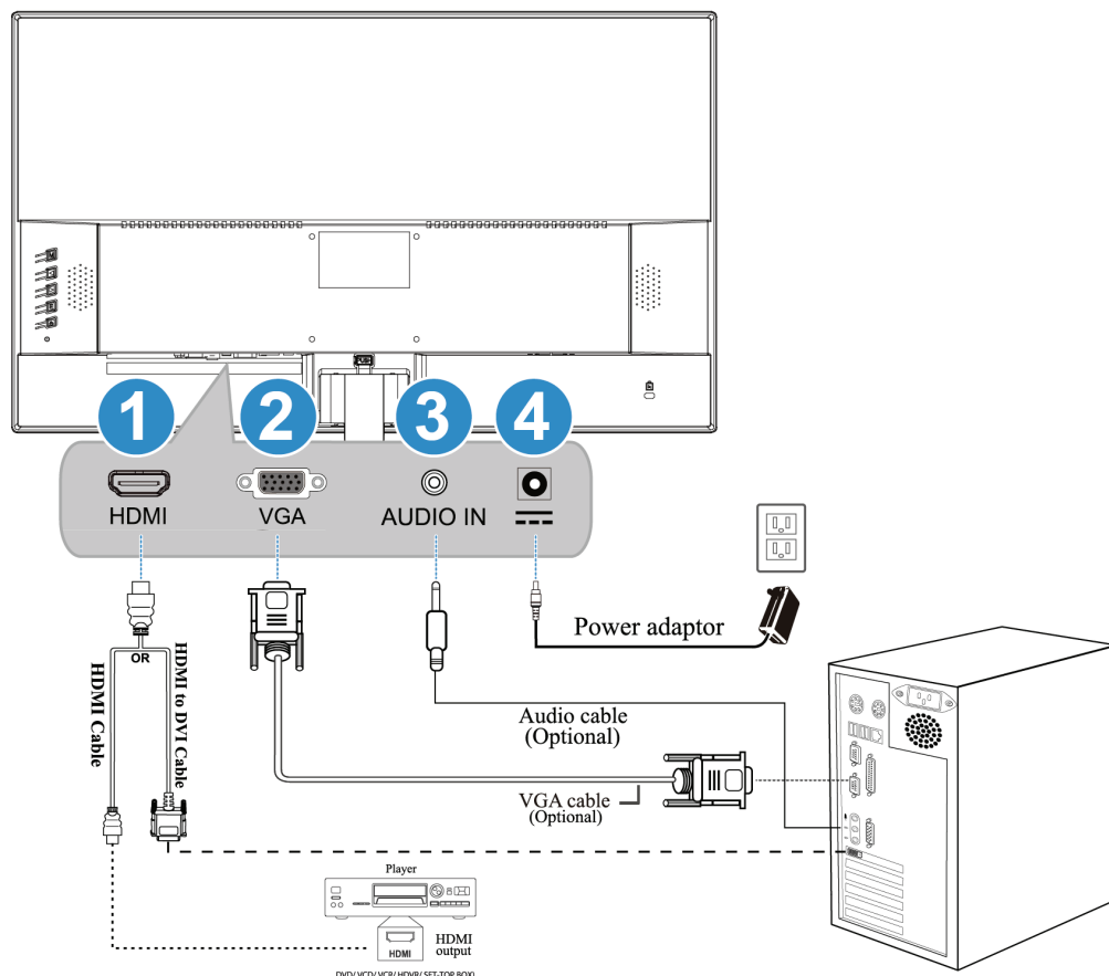
Figura 2. Branchement à un pc
