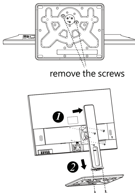
Figura.1. Installazione e Rimozione della Base
